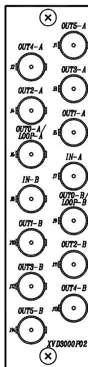
VISTA TRASERA DEL MODULO DVB3000
