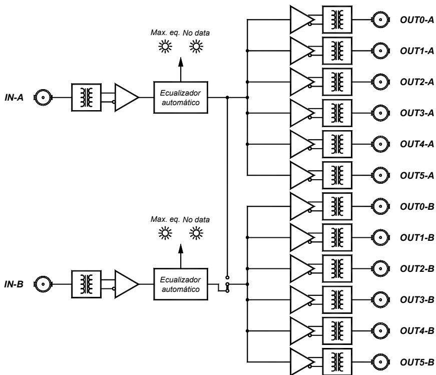
DIAGRAMA DE BLOQUES DEL DVB3000
